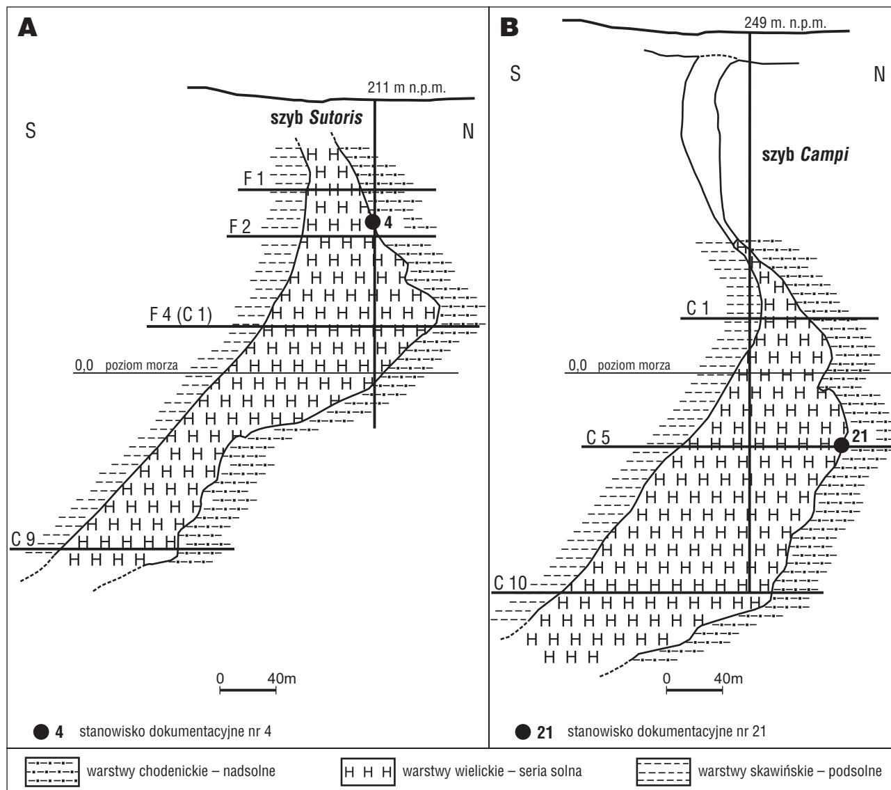
Ryc. 4. Lokalizacja wnioskowanego hipostatotypu warstw chodenickich (stanowiska dokumentacyjne nr 4 i 21) na tle schematycznego przekroju geologicznego złoża soli Bochnia (wg Poborskiego, 1952, uproszczony)
