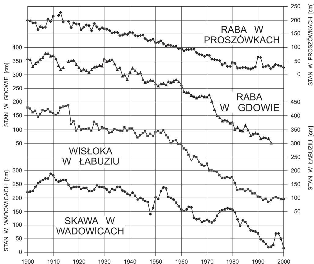
Ryc. 1.5. Zmiany minimalnych rocznych stanów Raby w posterunkach wodowskazowych Proszówki i Gdów, Wisłoki w posterunku Łabuzie i Skawy w posterunku Wadowice w ciągu XX wieku. Zróżnicowanie zmian minimalnych stanów wody w tych posterunkach ilustruje różnice przebiegu pogłębiania się koryt pomiędzy rzekami o małej (Wisłoka w Łabuziu) i dużej energii (Skawa w Wadowicach) oraz pomiędzy odcinkami danej rzeki o małej (Raba w Proszówkach) i dużej energii (Raba w Gdowie).
