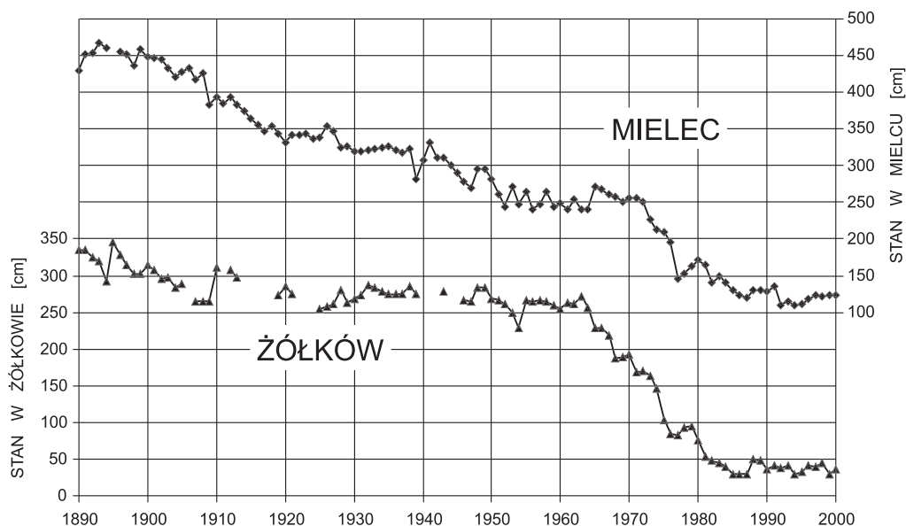
Ryc. 1.7. Zmiany minimalnych rocznych stanów Wisłoki w posterunku wodowskazowym Mielec w dolnym biegu rzeki oraz w posterunku Żółków w jej górnym biegu od 1890 roku.
