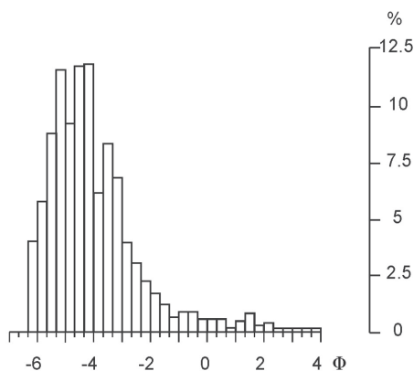
Ryc. 1.3. Żwiry łach środkowej Raby i histogramy ich uziarnienia (w procentach wagowych): (A) masywne żwiry o luźnym upakowaniu z drugiej połowy XIX wieku, o bimodalnym rozkładzie uziarnienia; (B) unimodalne żwiry niewypełnione z lat 50. XX wieku. Wielkość ziarna osadów przedstawiono w jednostkach \Phi . Poziomą szrafurą przedstawiono nierozdzielone frakcje najdrobniejsze.
